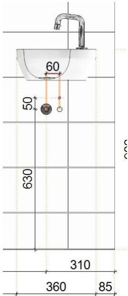
afvoer/toevoer fontein
